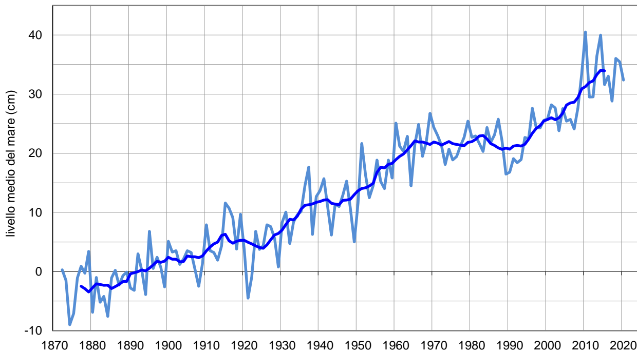
Figura 1 - Livello medio del mare a Venezia dal 1872 al 2020 e media mobile su 11 anni (dal 2020, nelle giornate di azionamento del MoSE, il l.m.m. giornaliero di Punta della Salute è integrato con quello di Piattaforma "Acqua alta")
