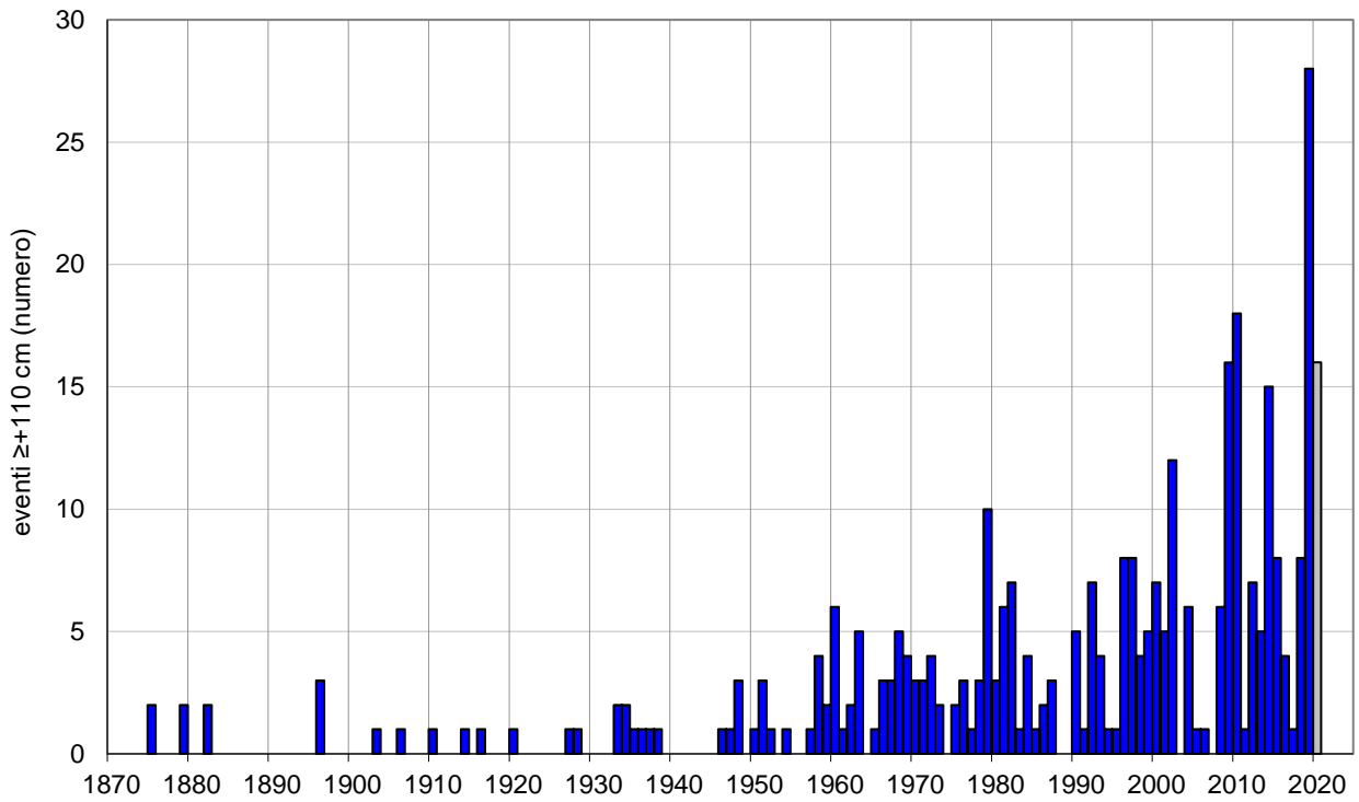
Figura 3 - Distribuzione annuale delle maree \geq +110 cm registrate a Venezia dal 1872 al 2019 (barra blu) e nel Golfo di Venezia dal 2020 (barra grigia)
