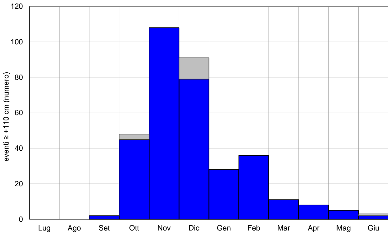
Figura 5 - Distribuzione mensile delle maree \geq +110 cm registrate dal 1872 al 2019 a Venezia (area blu) e dal 2020 nel Golfo di Venezia (area grigia)
