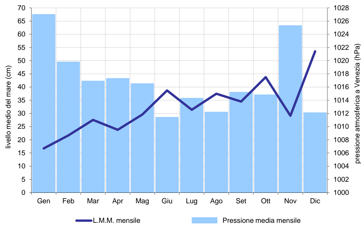
Figura 2 - Variazione del livello medio mare e della pressione media mensili nel 2020 (dal 2020, nelle giornate di azionamento del MoSE, il l.m.m. giornaliero di Punta della Salute è integrato con quello di Piattaforma "Acqua alta")
