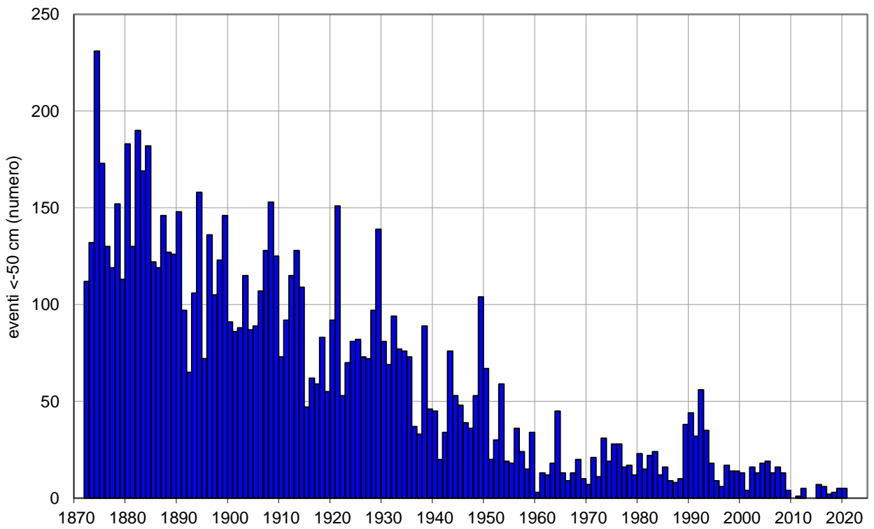
Figura 4 - Distribuzione annuale delle maree < -50 cm registrate a Venezia dal 1872 al 2020
