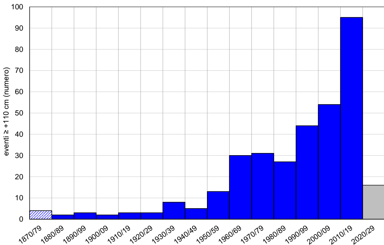
Figura 6 - Distribuzione decennale delle maree \geq +110 cm registrate dal 1872 al 2019 a Venezia (area blu) e dal 2020 nel Golfo di Venezia (area grigia)
